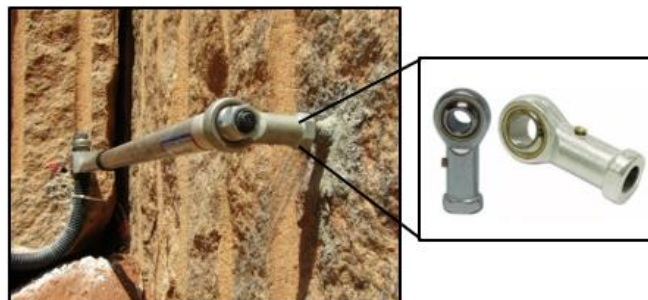
Figura 6. Método de instalação dos equipamentos.
